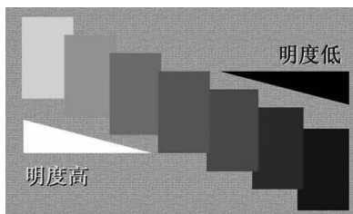
图 2-10 明度变化
